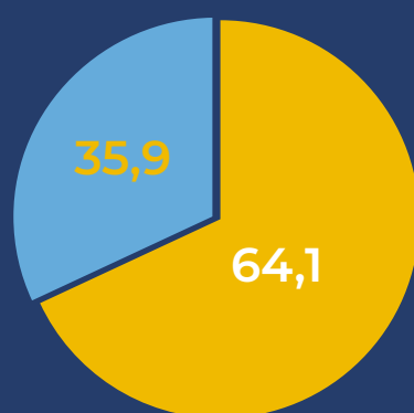
Pareto
